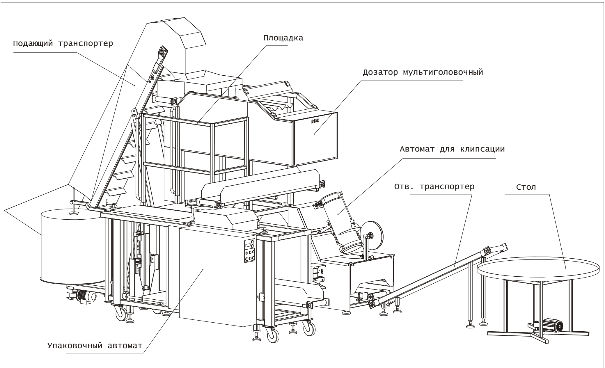
Автоматическая линии с двумя выходами
